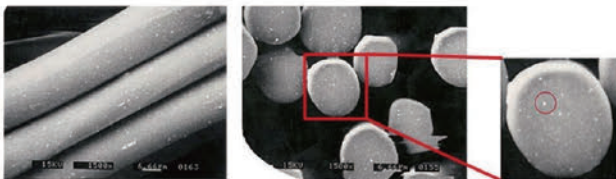
光電子が練り込まれた繊維の断面(断面の中の白い点が光電子セラミックス)
